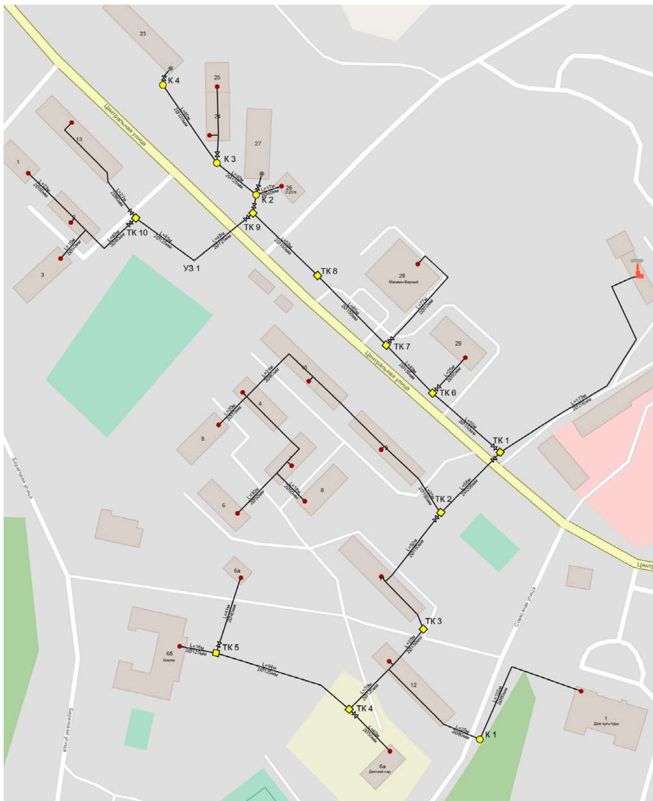
Рисунок 1.2. Карта (схема) тепловых сетей д. Раздолье по состоянию на 01.11.2021 г.
