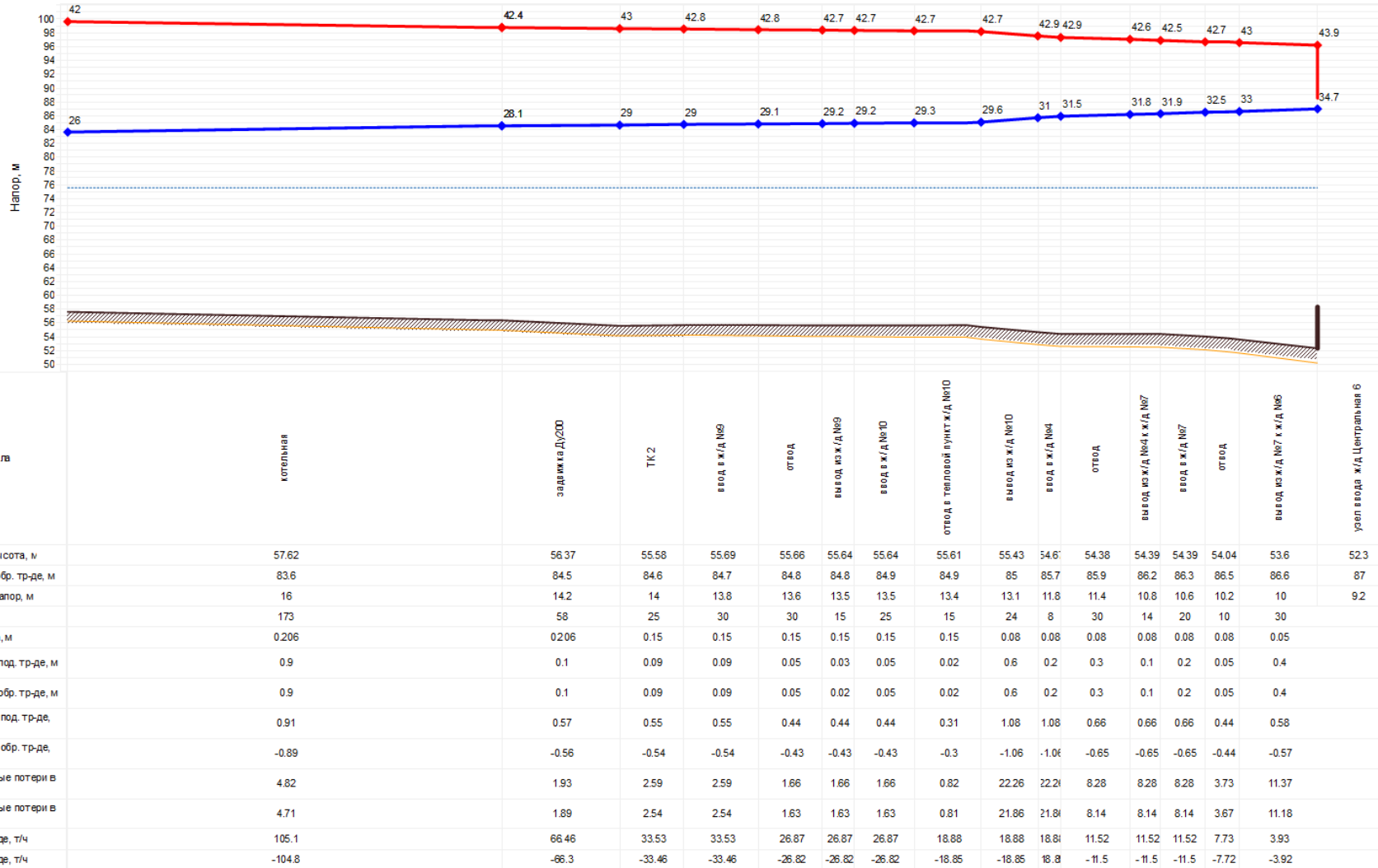
Рисунок 1.12. Пьезометрический график от котельной до узла ввода в жилой дом ул. Центральная, 6 (с учетом выполнения наладочных работ)
