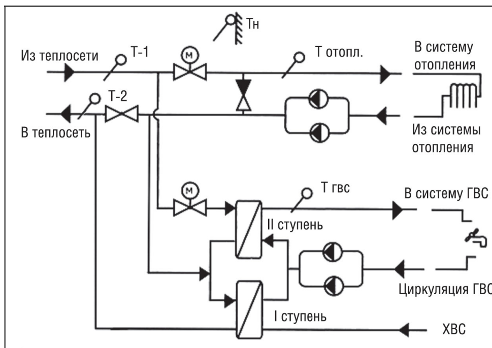
Рисунок 7.1.2. Присоединение ГВС по двухступенчатой схеме при зависимой схеме подключения системы отопления
