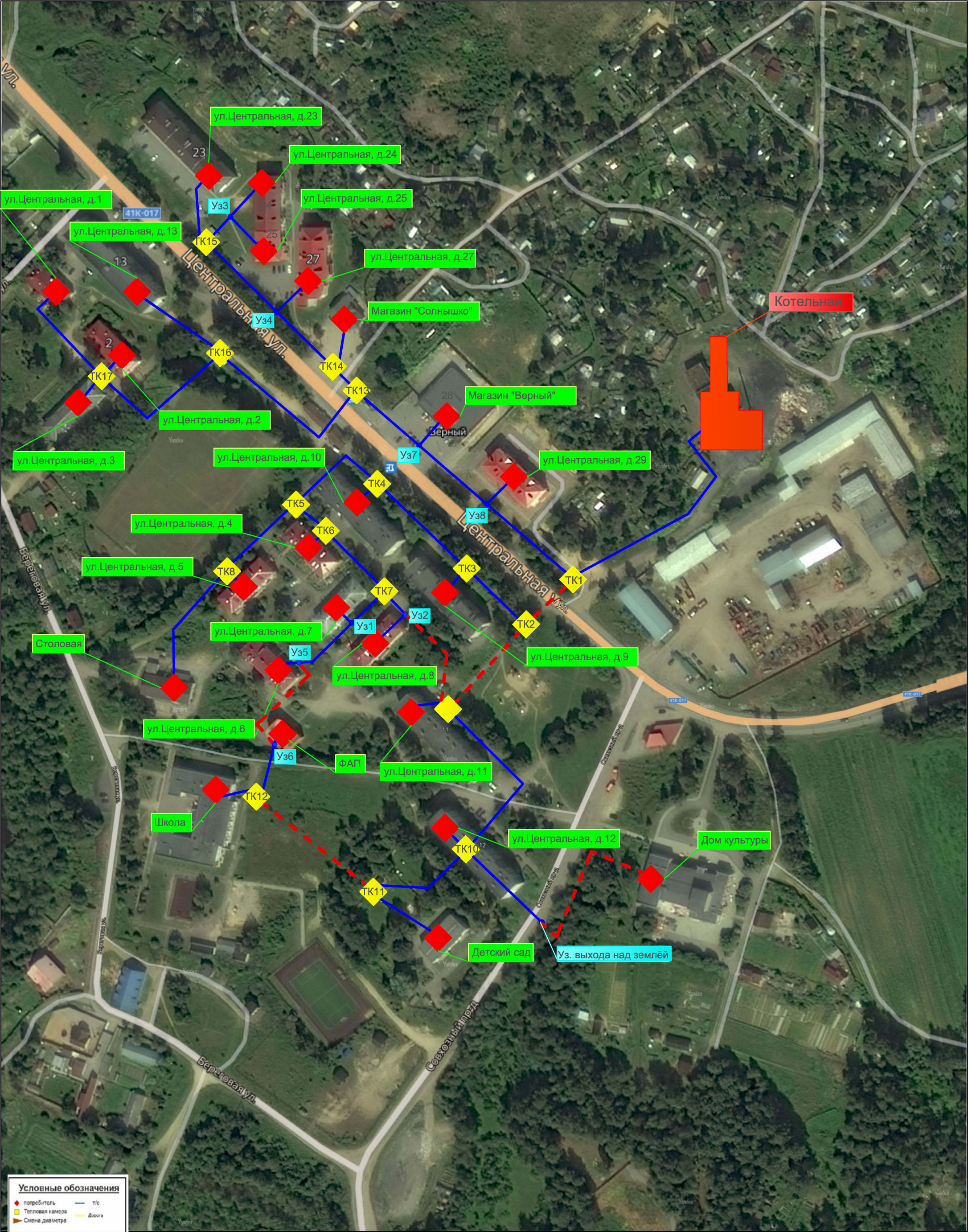
Рис. 6.3.1 Перспективная карта-схема тепловых сетей д. Раздолье
