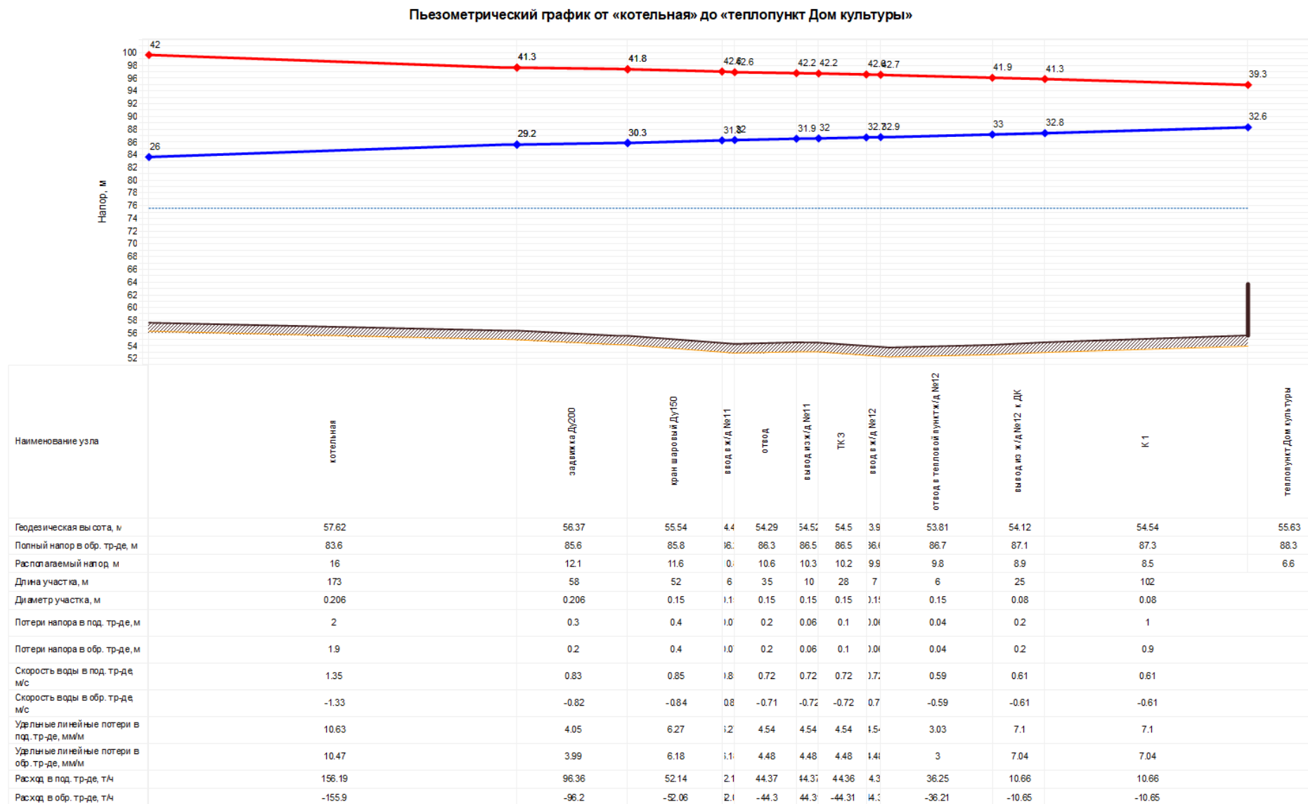
Рисунок 1.9. Пьезометрический график от котельной до индивидуального теплового пункта МУК «Раздольское клубное объединение» (фактический режим работы тепловых сетей)
