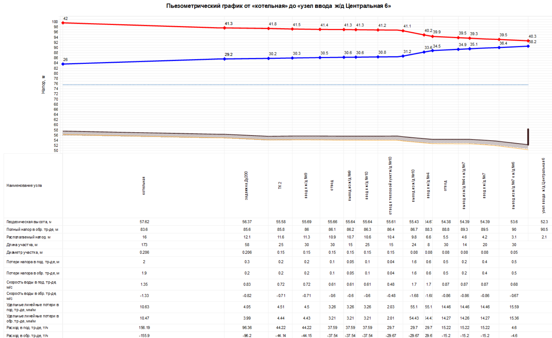
Рисунок 1.7. Пьезометрический график от котельной до узла ввода в жилой дом ул. Центральная, 6 (фактический режим работы тепловых сетей)
