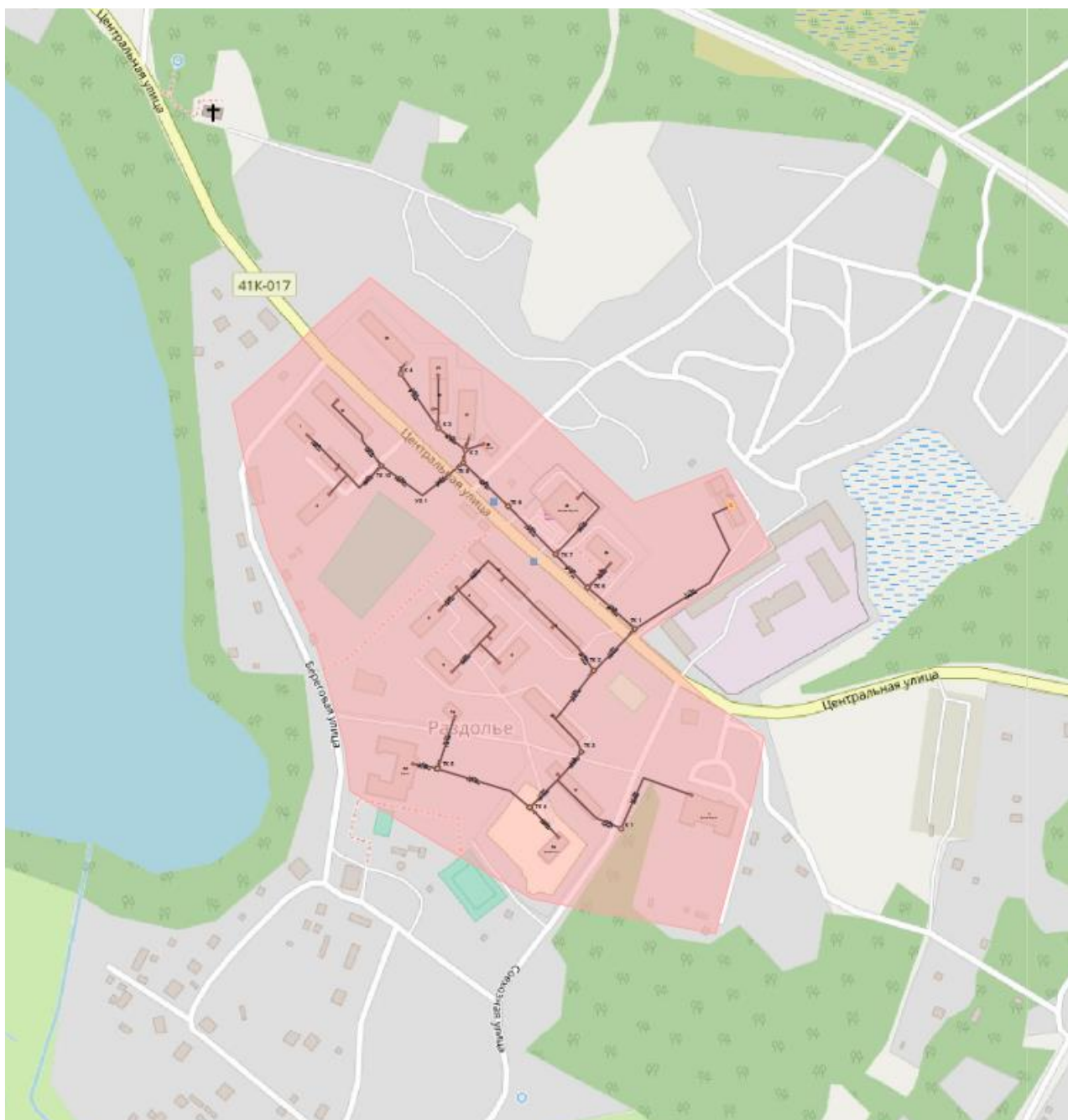
Рисунок 1.1. Зона действия централизованного источника теплоснабжения
