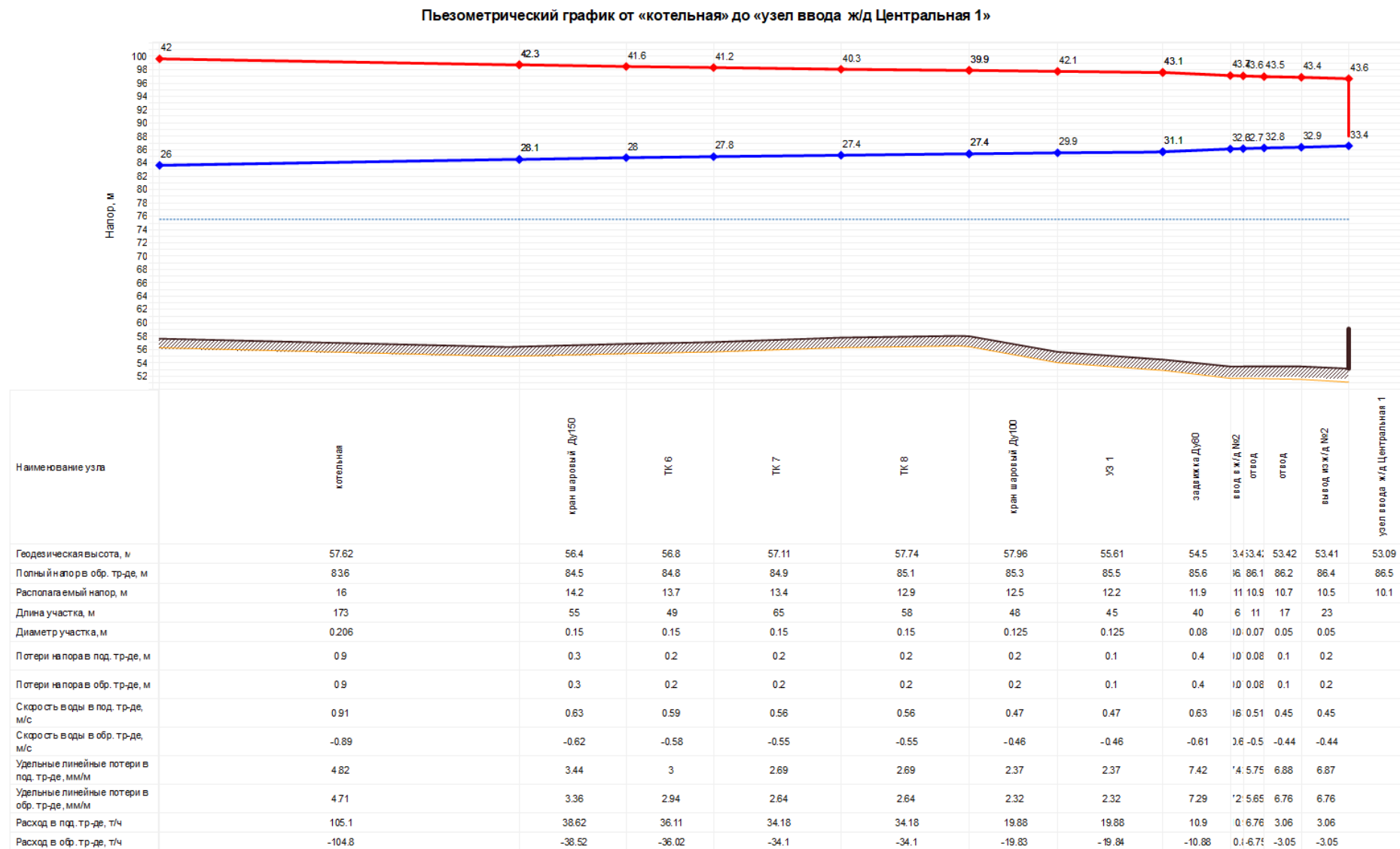
Рисунок 1.10. Пьезометрический график от котельной до узла ввода в жилой дом ул. Центральная, 1 (с учетом выполнения наладочных работ)
