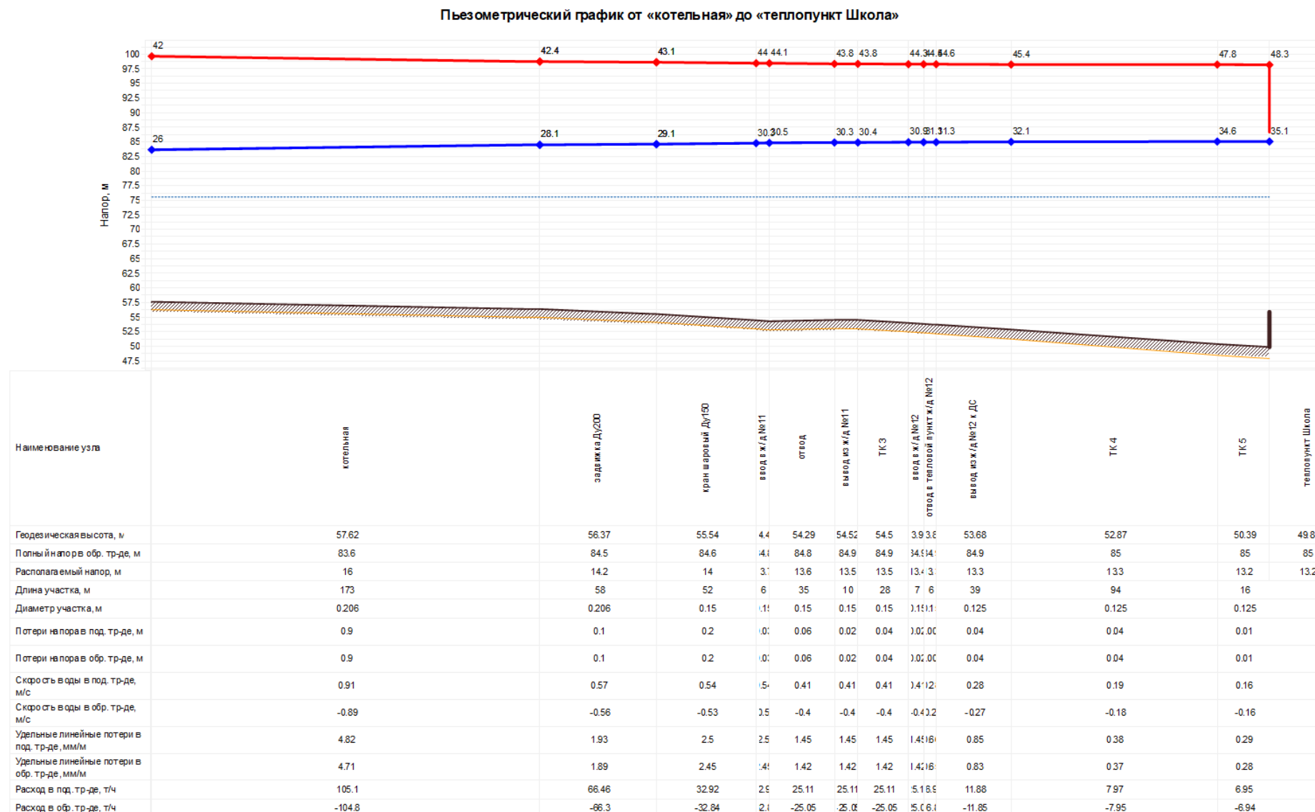
Рисунок 1.13. Пьезометрический график от котельной до индивидуального теплового пункта МОУ «Раздольская СОШ» (с учетом выполнения наладочных работ)
