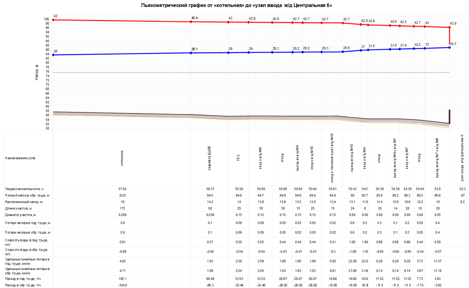
Рисунок 1.12. Пьезометрический график от котельной до узла ввода в жилой дом ул. Центральная, 6 (с учетом выполнения наладочных работ)
