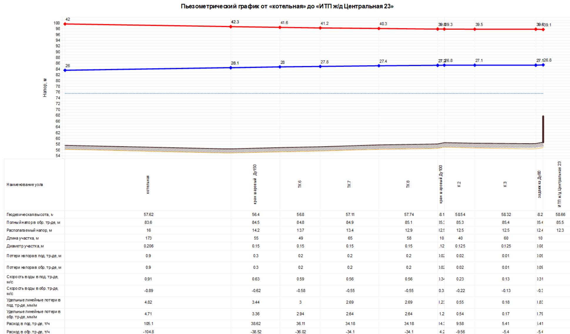
Рисунок 1.11. Пьезометрический график от котельной до индивидуального теплового пункта жилого дома ул. Центральная, 23 (с учетом выполнения наладочных работ)
