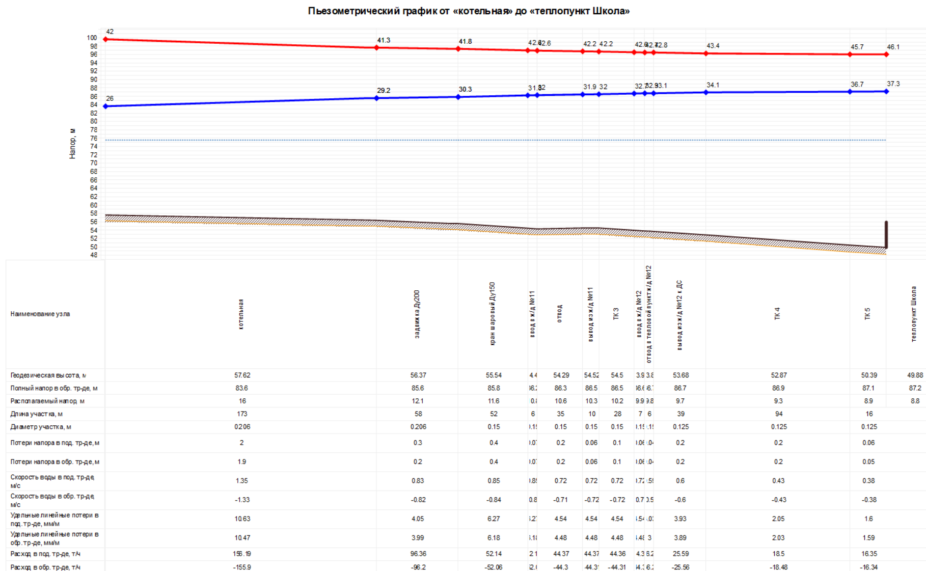
Рисунок 1.8. Пьезометрический график от котельной до индивидуального теплового пункта МОУ «Раздольская СОШ» (фактический режим работы тепловых сетей)
