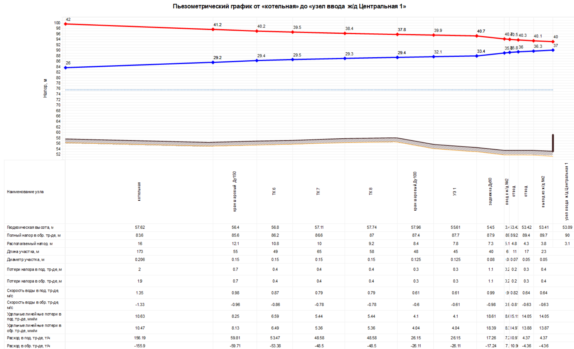
Рисунок 1.5. Пьезометрический график от котельной до узла ввода в жилой дом ул. Центральная, 1 (фактический режим работы тепловых сетей)
