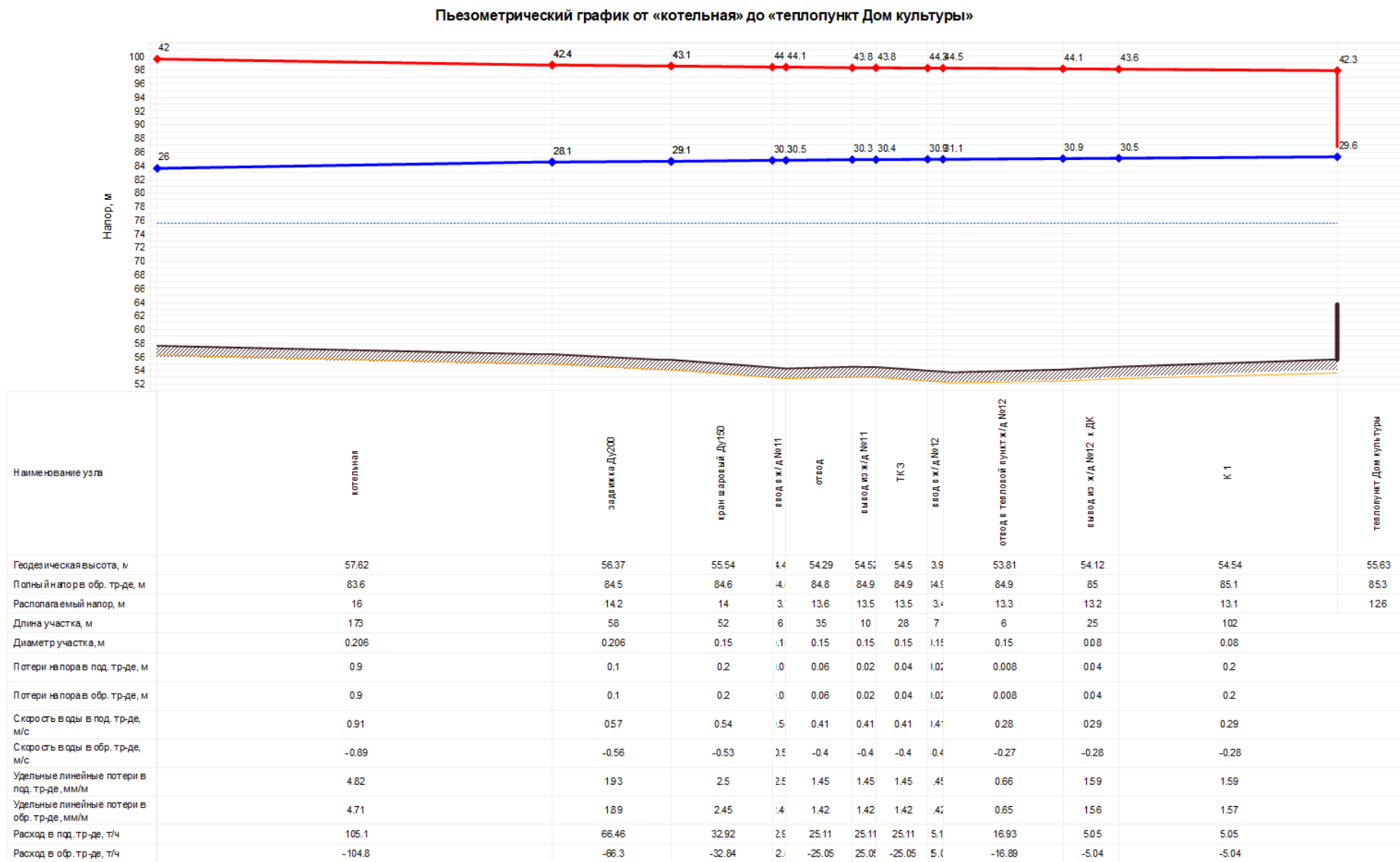
Рисунок 1.14. Пьезометрический график от котельной до индивидуального теплового пункта МУК «Раздольское клубное объединение» (с учетом выполнения наладочных работ)
